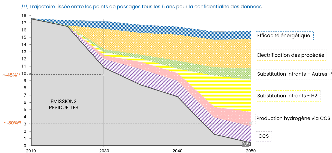
EVOLUTION DES ÉMISSIONS FOSSILES DES INDUSTRIELS EXISTANTS par levier de décarbonation Illustration basée sur le scénario AMBITIEUX
